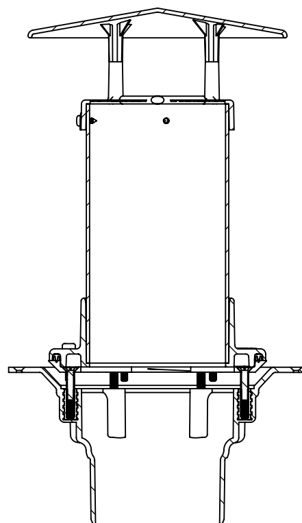
SECTION AA-AA
