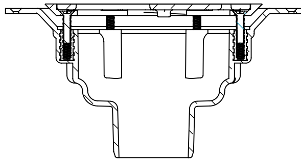
SECTION D-D
