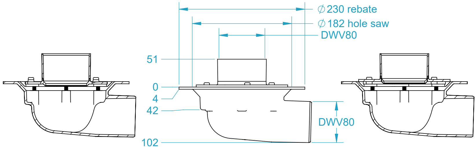
SECTION AK-AK
