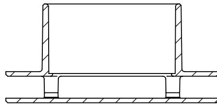
SECTION D-D
