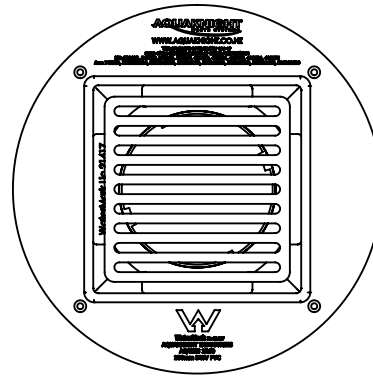
Slotted Lid 4000.155
