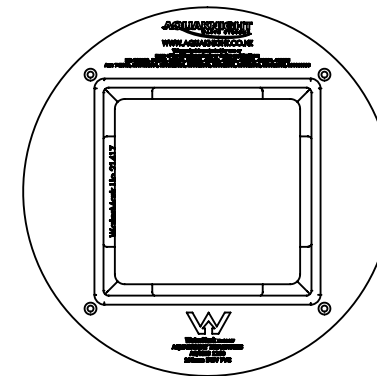
4000.143 Solid Lid
