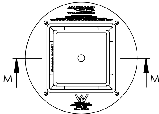
4000.144 Tile Insert
