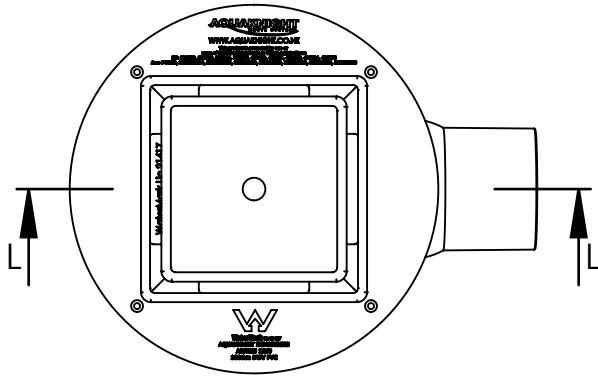
4000.104 Tile Insert
