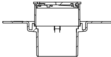
SECTION J-J SCALE 1 : 4
