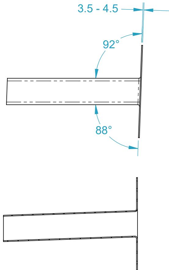
SECTION A-A
