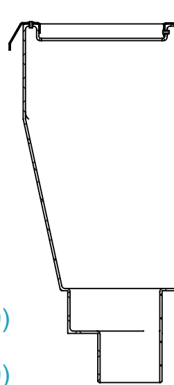
SECTION A-A
